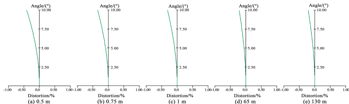
图 7 波前编码系统的畸变
