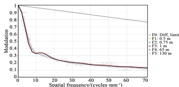
(b) 波前编码系统 MTF 曲线
